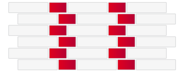
ГОТИЧЕСКАЯ КЛАДКА
