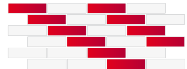
ЛОЖКОВАЯ КЛАДКА СДВИГ НА 1/4 КИРПИЧА
