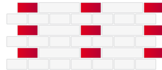
ГОЛЛАНДСКАЯ КЛАДКА
